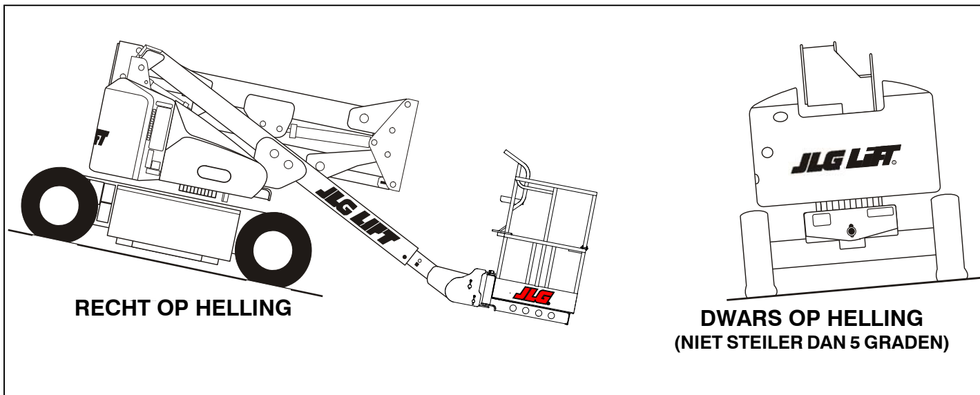
Figuur 4-3. Recht en dwars op helling
