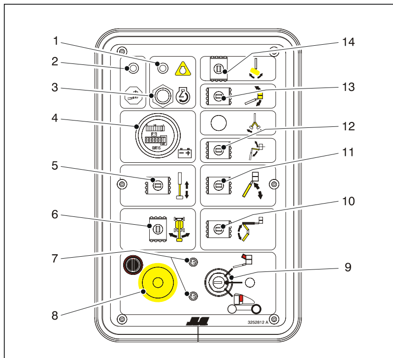
Figuur 3-1. Grondbedieningsstation
